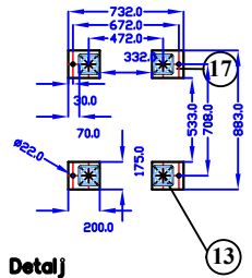
Rastojanje otvora za ankerisanje
